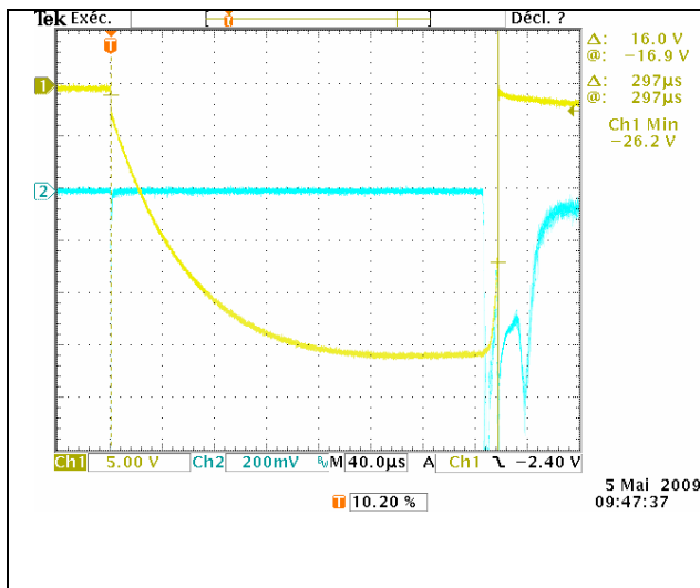
Enregistrement du choc n°16 (Tek00) [1] : Forme d'onde de tension [2] : Lumière UV émise par la décharge
