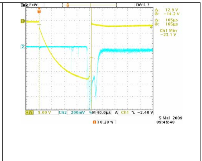
Enregistrement du choc n°17 (Tek01) [1] : Forme d'onde de tension [2] : Lumière UV émise par la décharge
